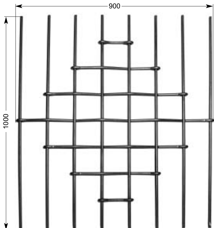
26 453* 11,00 kg Ø 12 mm
