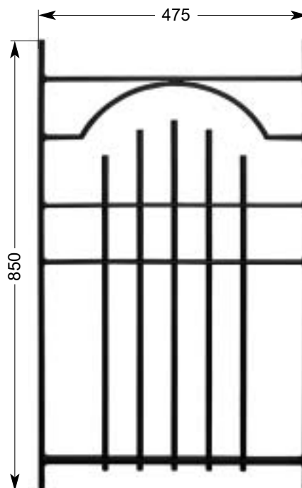
22 712 8,50 kg Ø 12 mm □ 20 x 10 mm
