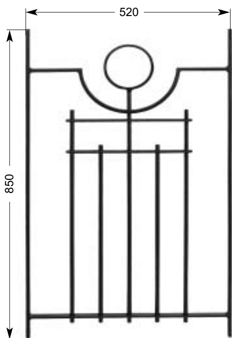
22 710 7,50 kg Ø 12 mm □ 20 x 10 mm
