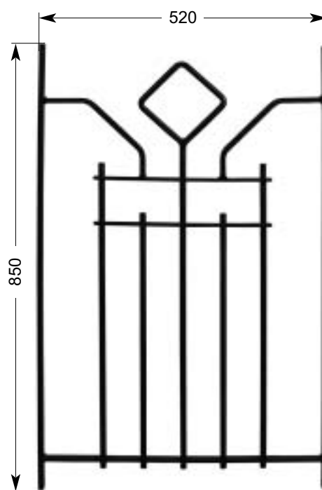
22 711 7,50 kg Ø 12 mm □ 20 x 10 mm
