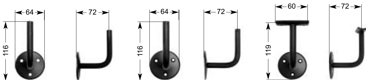
17 619 0,21 kg Ø 12 mm ⊙ 3 x 6,5 mm
