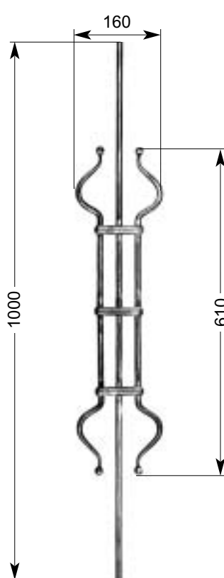
36 413 2,23 kg Ø 12 mm
