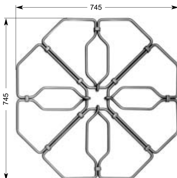
26 444 7,37 kg Ø 12 mm
