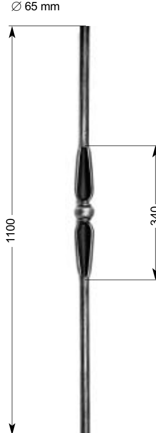
30 307 Anfangsstab mit Messingkugel Endpost with brass ball Balustre de départ boule en laiton 4,72 kg Ø 25 mm
