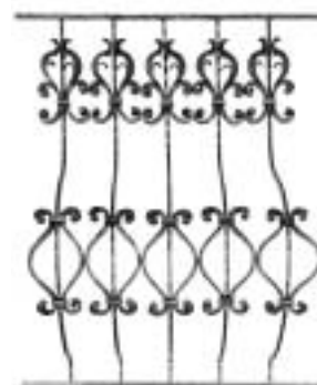
32 402 Korbstab Convex grille bar Barreaux de grille en anse-de-panier 2,76 kg □ 16 x 8 mm
