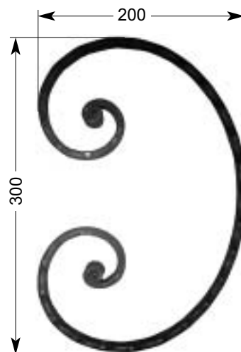
25 403 0,87 kg □ 16 x 8 mm
