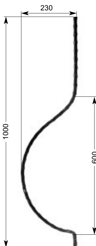
32 401 Korbstab Convex grille bar Barreaux de grille en anse-de-panier 0,97 kg □ 16 x 8 mm
