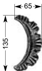
25 501 0,11 kg □ 3,5 mm passend zu suitable to approprié 25 401
