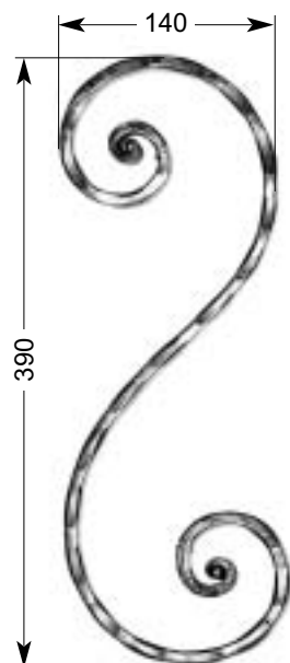
25 461 0,79 kg □ 16 x 8 mm
