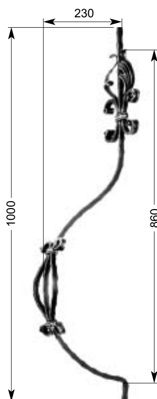
32 402 Korbstab Convex grille bar Barreaux de grille en anse-de-panier 2,76 kg □ 16 x 8 mm
