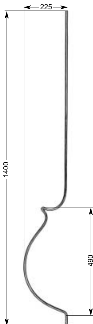
32 121 Korbstab Convex grille bar Barreaux de grille en anse-de-panier 1,95 kg Ø 14 mm
