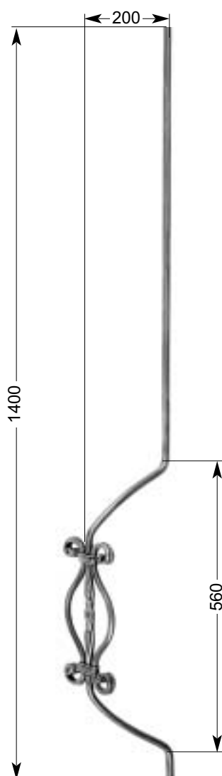
32 144 Korbstab Convex grille bar Barreaux de grille en anse-de-panier 2,87 kg Ø 14 mm
