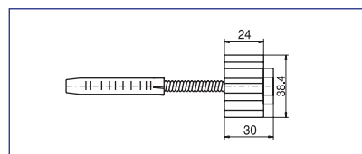
78 222 Wandanschluß PE-Zapfen für 42,4 x 2 mm Edelstahlschraube und Dübel Ø 10 mm 0,05 kg Wall connection with PE-attachment for 42,4 x 2 mm with inox screw and dowel 10 mm Fixation de paroi avec PE- approche pour 42,4 x 2 mm avec vis en inox et cheville 10 mm
