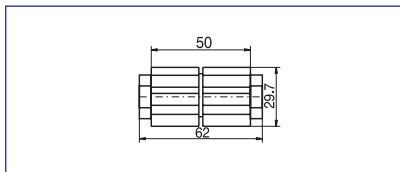
78 121 PE-Rohrverbinder für 33,7 x 2 mm 0,05 kg PE-connection for 33,7 x 2 mm Lien de tube en PE pour 33,7 x 2 mm
