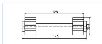
78 223 Rohrverbinder zum Biegen mit PE-Zapfen für 42,4 x 2 mm 0,13 kg Tube connection for bending with PE-attachment for 42,4 x 2 mm Lien de tube pour plier avec PE- approche pour 42,4 x 2 mm
