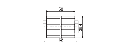
78 221 PE-Rohrverbinder für 42,4 x 2 mm 0,06 kg PE-connection for 42,4 x 2 mm Lien de tube en PE pour 42,4 x 2 mm
