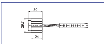
78 122 Wandanschluß PE-Zapfen für 33,7 x 2 mm Edelstahlschraube und Dübel Ø 10 mm 0,04 kg Wall connection with PE-attachment for 33,7 x 2 mm with inox screw and dowel 10 mm Fixation de paroi avec PE- approche pour 33,7 x 2 mm avec vis en inox et cheville 10 mm
